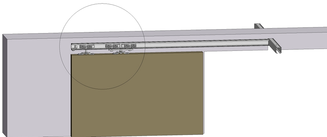
Detalje af løbevogne og beslag over dørbladet
